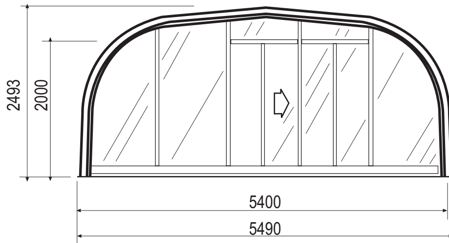
FACHADA FIJA - 1 PUERTA CENTRO VISTA EXTERIOR
